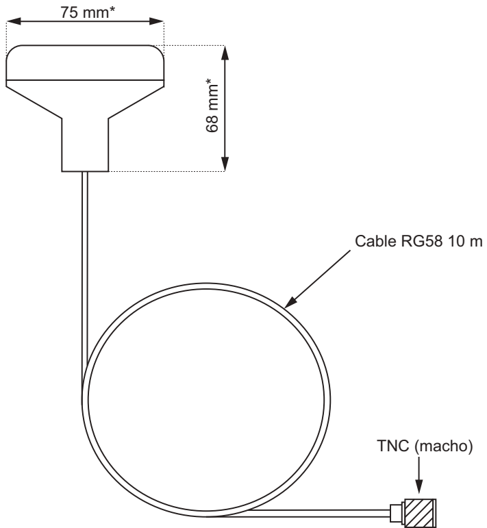
Figura 31 Antena GNSS
