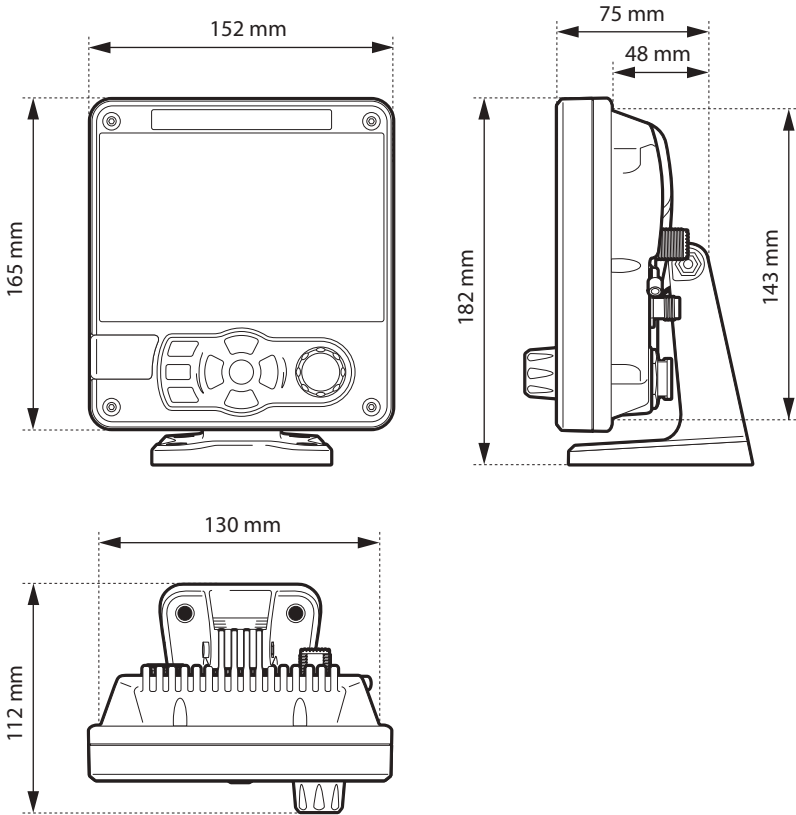
Figura 30 Dimensiones del transceptor AIS
