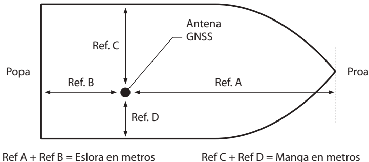
Figura 22 Medición de las dimensiones de la embarcación
