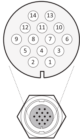
Figura 12 Conexiones del cableado del conector de 14 vías
